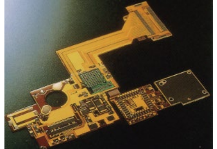
FPC (フレキシブルプリントサーキット)
